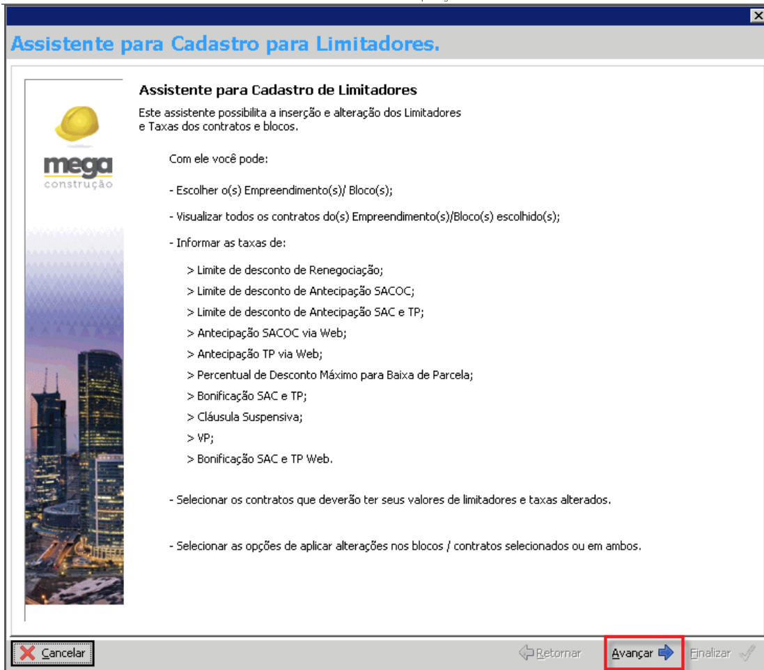
Assistente para cadastro de limitadores
